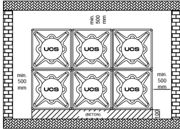
BETON ÜST GÖRÜNÜŞÜ / CONCRETE BASE TOP-APPEARANCE
